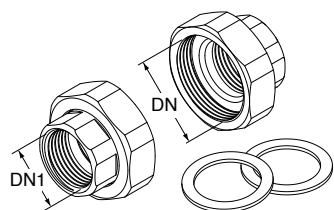
Raccords d'adaptation en fonte
